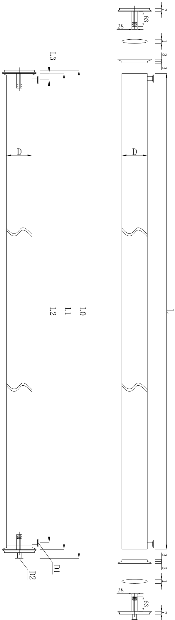
4英寸3芯膜壳图纸
