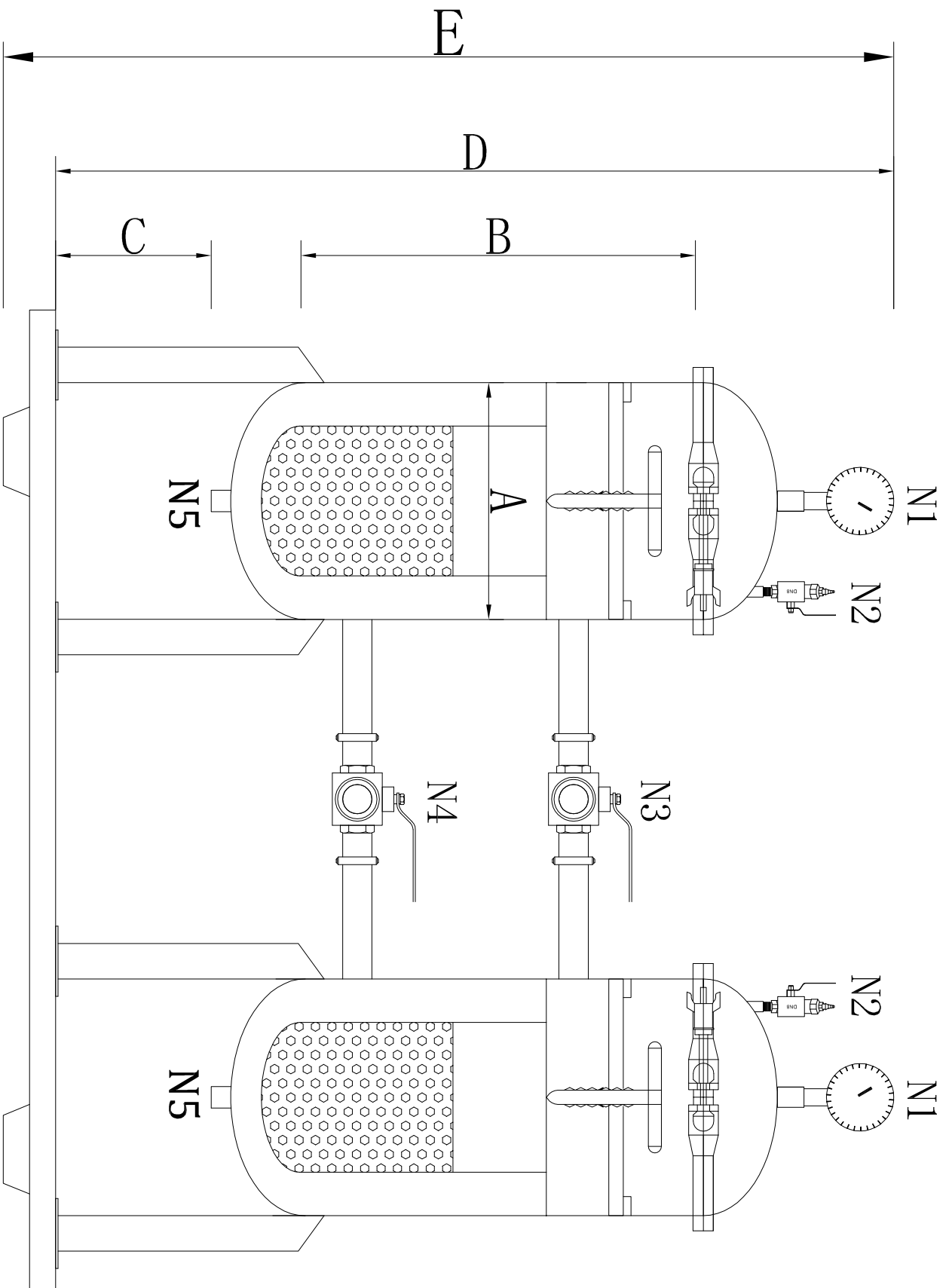
侧视图
